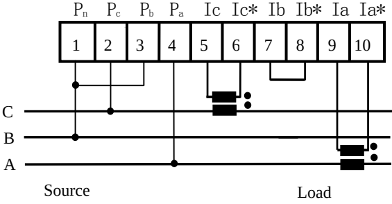
(2) 三相三线不平衡负载 (3P3W)
