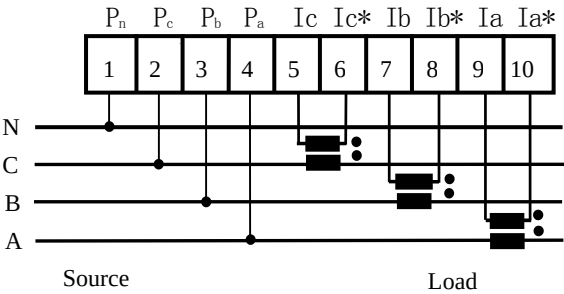
(1) 三相四线不平衡负载 (3P4W)
